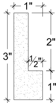
SCALE: 6" - 1"
