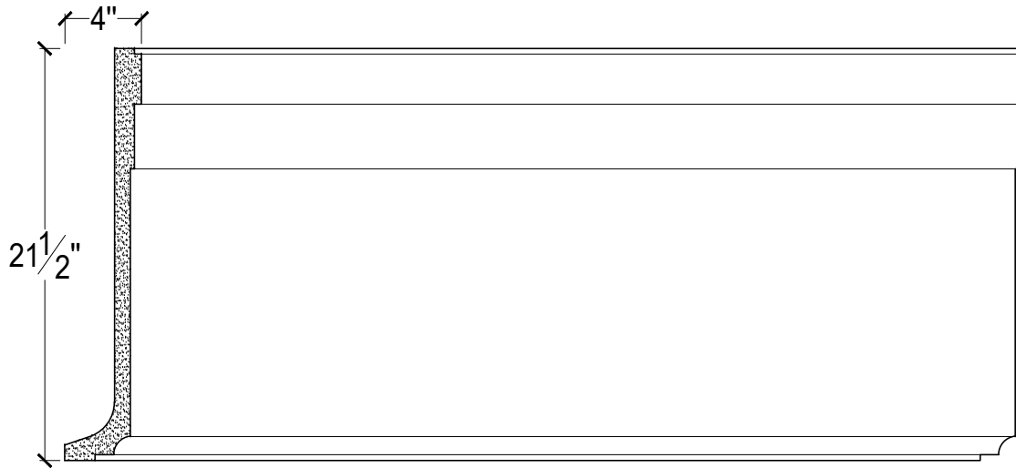
SCALE :7"=1'
