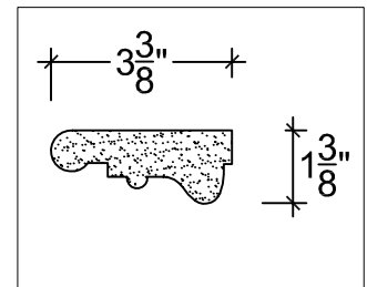
SECTION SCALE: 3" = 1'
