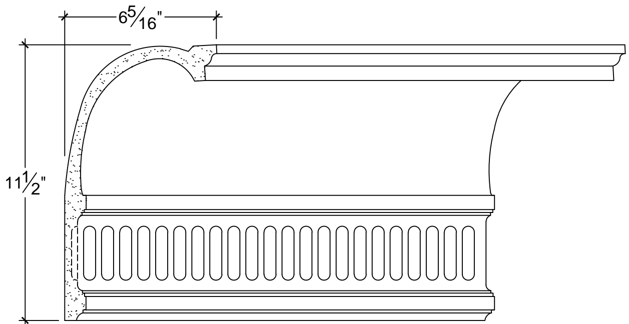
SCALE: 3" = 1'
