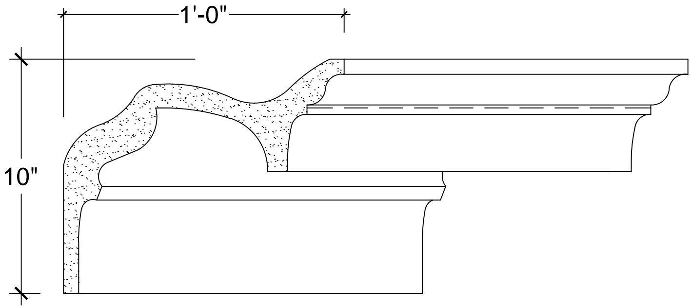
SCALE: 3" - 1"
