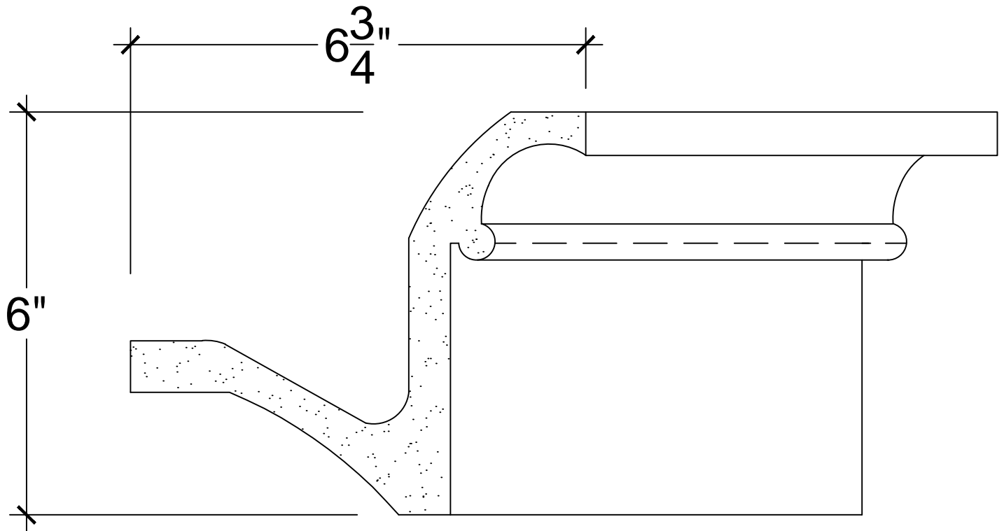
SCALE: 6" - 1"
