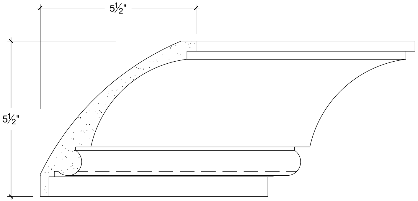
SCALE: 6" = 1'-0"
