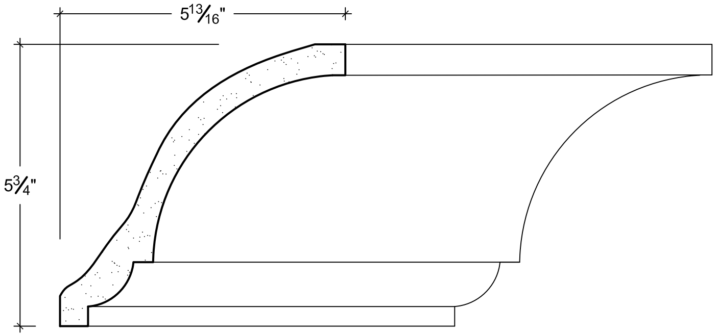
SCALE: 6" = 1'
