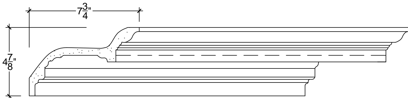
SCALE: 3" - 1"
