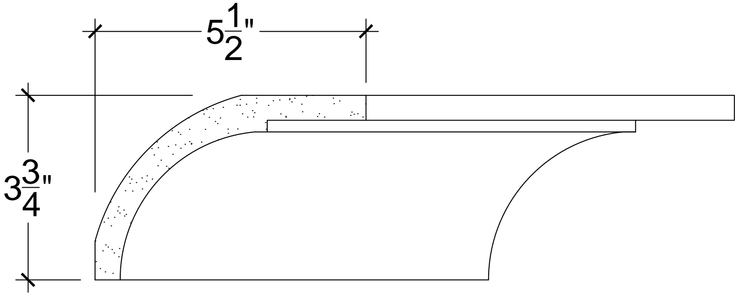
SCALE: 6" - 1'-0"
